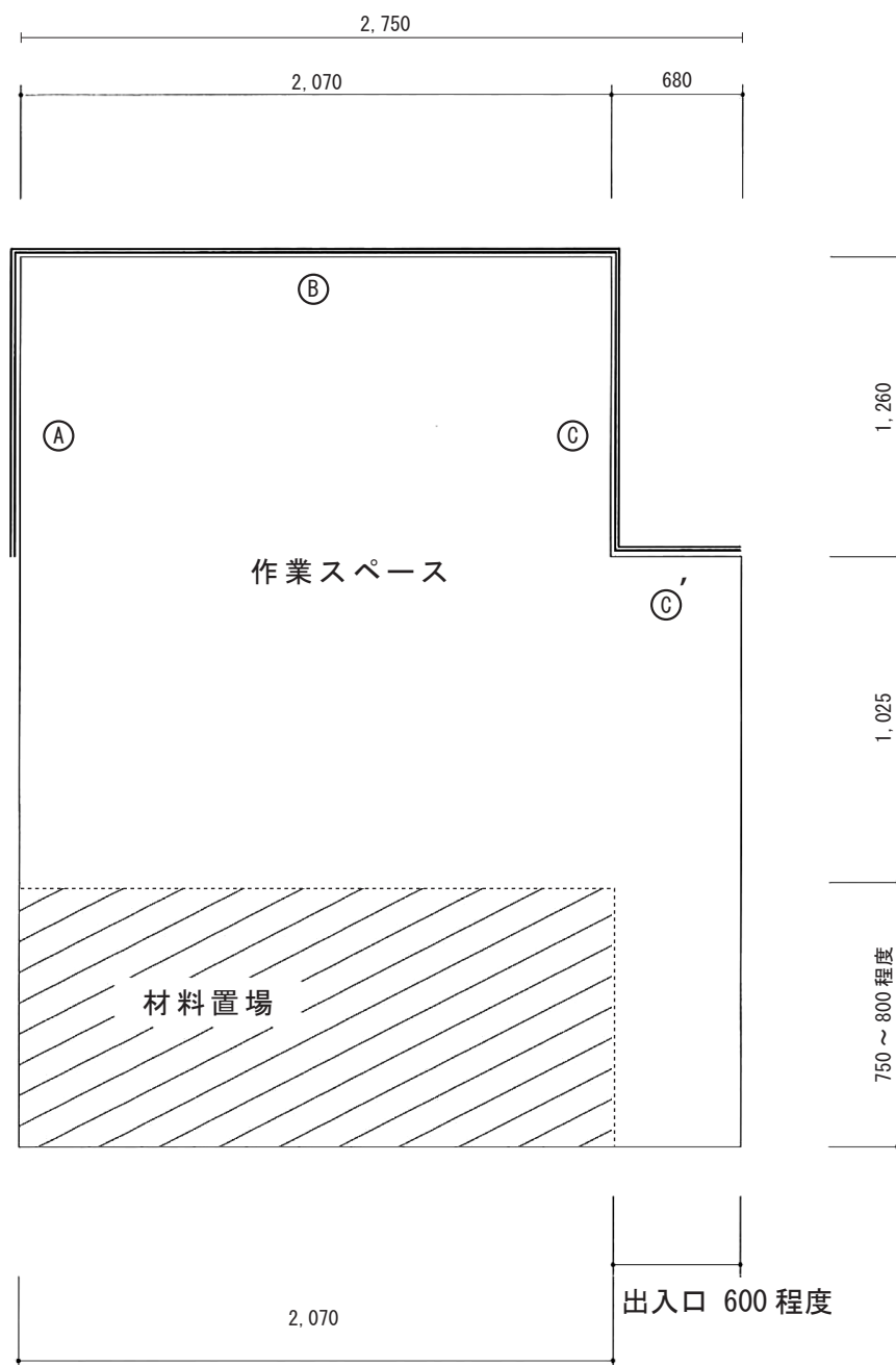
選手1人分 作業スペース図
